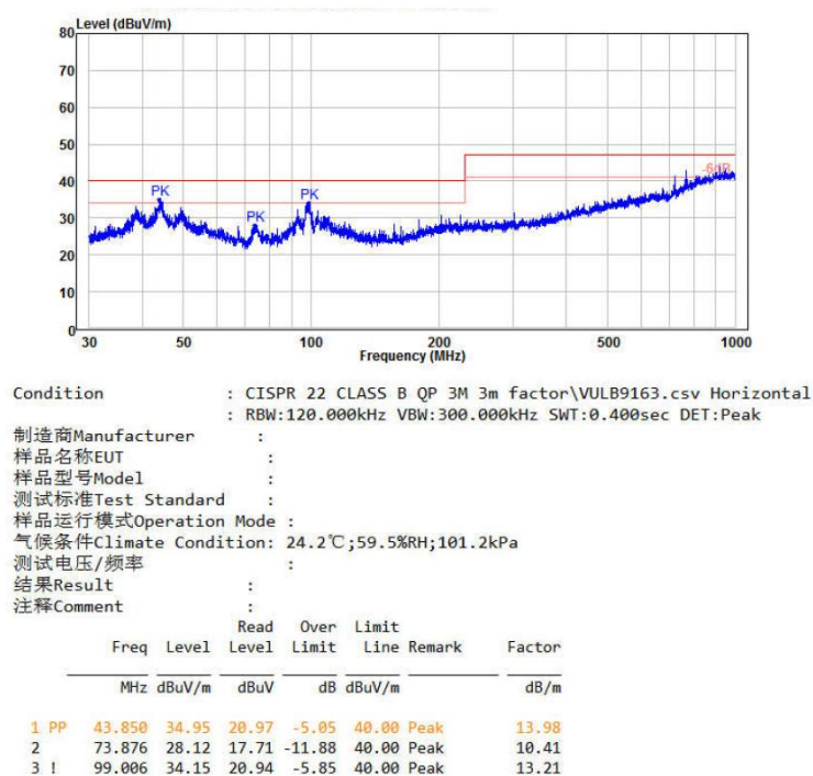
图 5-7 辐射测试垂直方向
