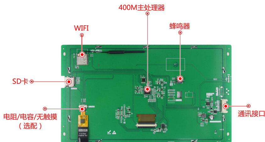
图 1-4 硬件配置图
