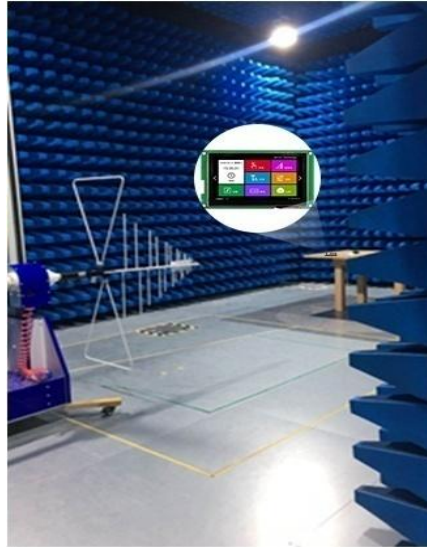
图 5-5 辐射测试图
