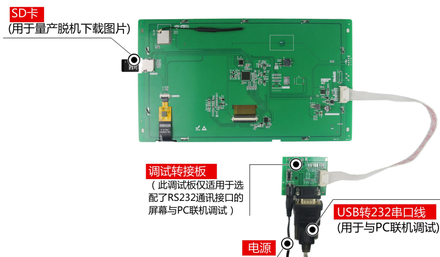
图 1-5 调试工具图
