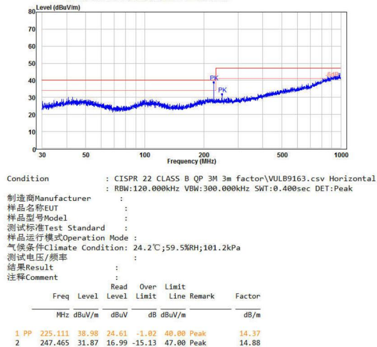
图 5-6 辐射测试水平方向
